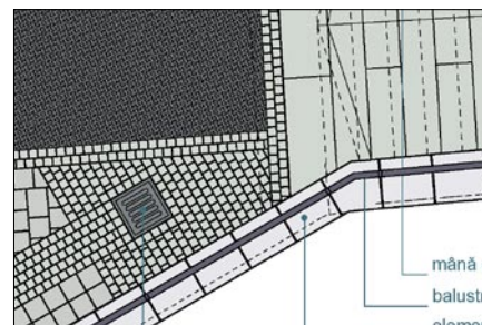
Detalii de pavaj, Terasa Soarelui, Sibiu
