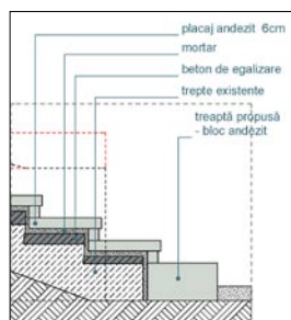
PUD Parcaj supraterean etajat, str. Moșilor, Cluj
